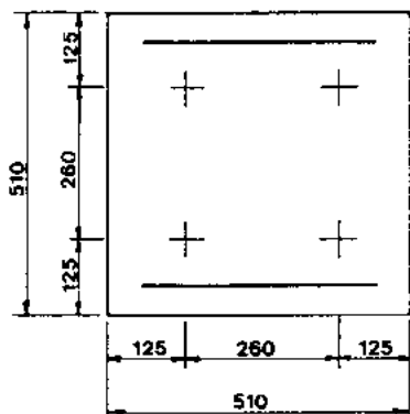
KRONE FOR 4 STK. SØYLER VEKT: 54 kg
