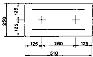
KRONE FOR 2 STK. SØYLER VEKT: 27 kg
